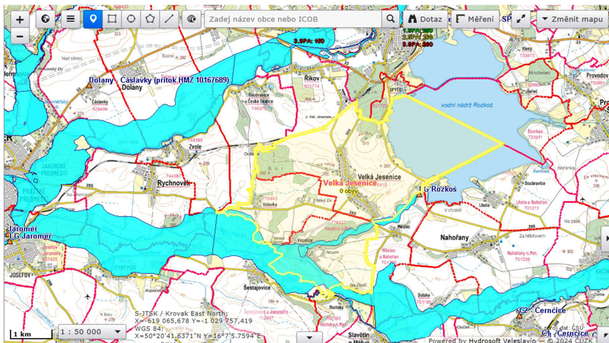
Obrázek 4: Záplavová území
